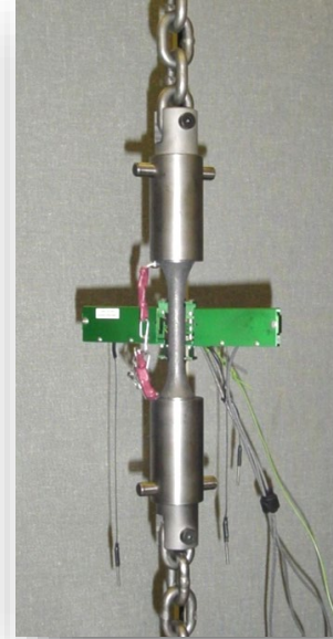
Tensile Strength
